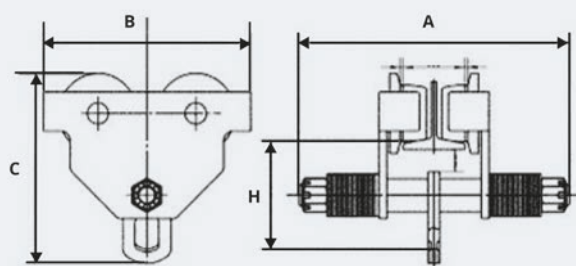
CARRELLI PER PUTRELLA
