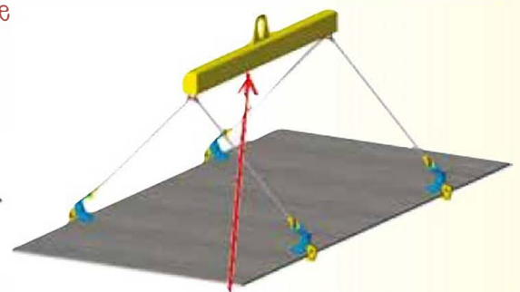
per lastre lunghe usare barra distanziatrice (bilancino)
